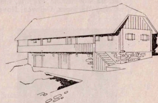
Slika 56. Vrhlevna kmetijska hiša v Pančgrčgrmu v Gorjanskem Podgorju. Spodaj sta hlev in kevder, zgoraj pa stanovanjski prostori z značilnim simetričnim ustrojem. Pred hišo na dvorišču je gnojišče. Pri njej občudujemo razumno uporabljene višinske razlike tal, neustrezni pa so higienski pogoji zaradi namestitve hleva pod stanovanjem in zaradi nevarovanega gnojišča pred hišo.
