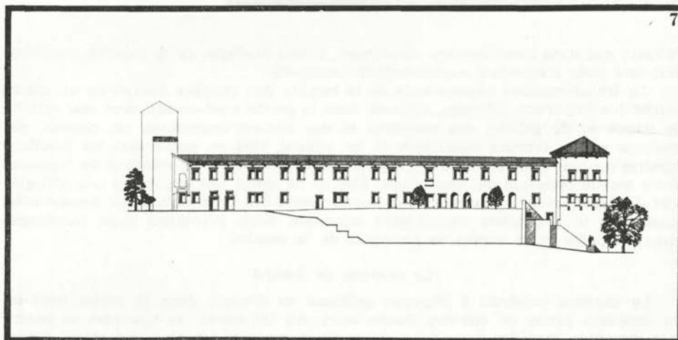
Projekta za rekonstrukcijo grajske dvoriščne fasade in fasade zgornjega grajskega trakta. — Projekt. ing. N. Sumi Projets pour la reconstruction de la façade du château donnant sur la cour et de la façade de l'aile supérieure du château. — Projets de l'ing. N. Sumi
